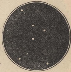
Una porción de cielo estrellado, á simple vista.
